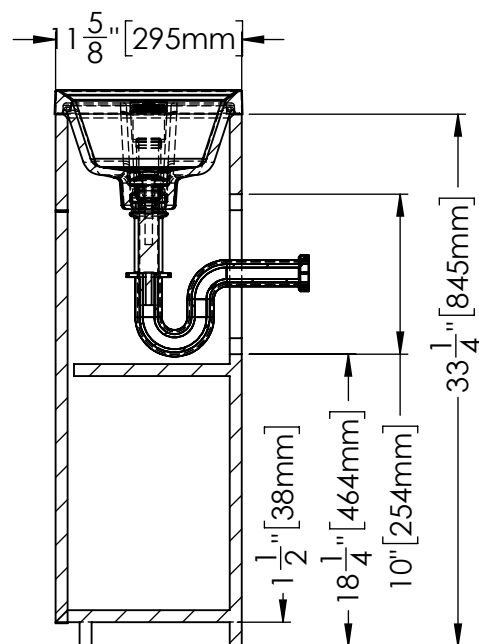
SECTION D-D
